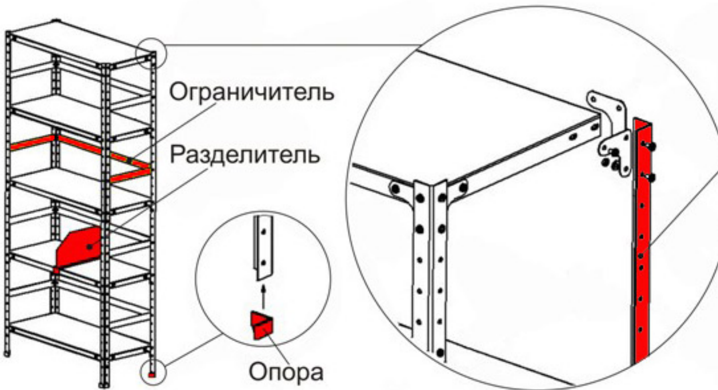
Полка (Dh-7005) с двумя полками, двумя перегородками, двумя ограничителями и двумя опорами
